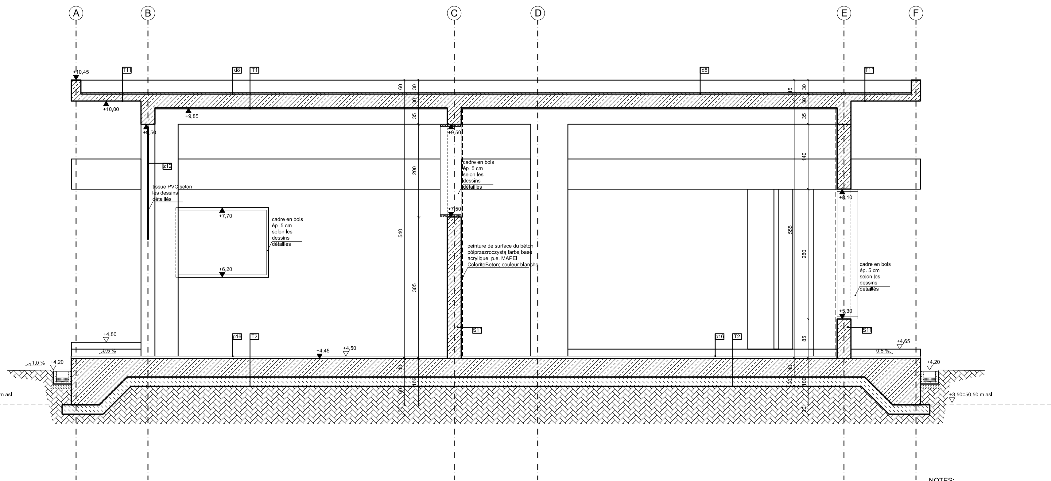
COUPE 21-22
