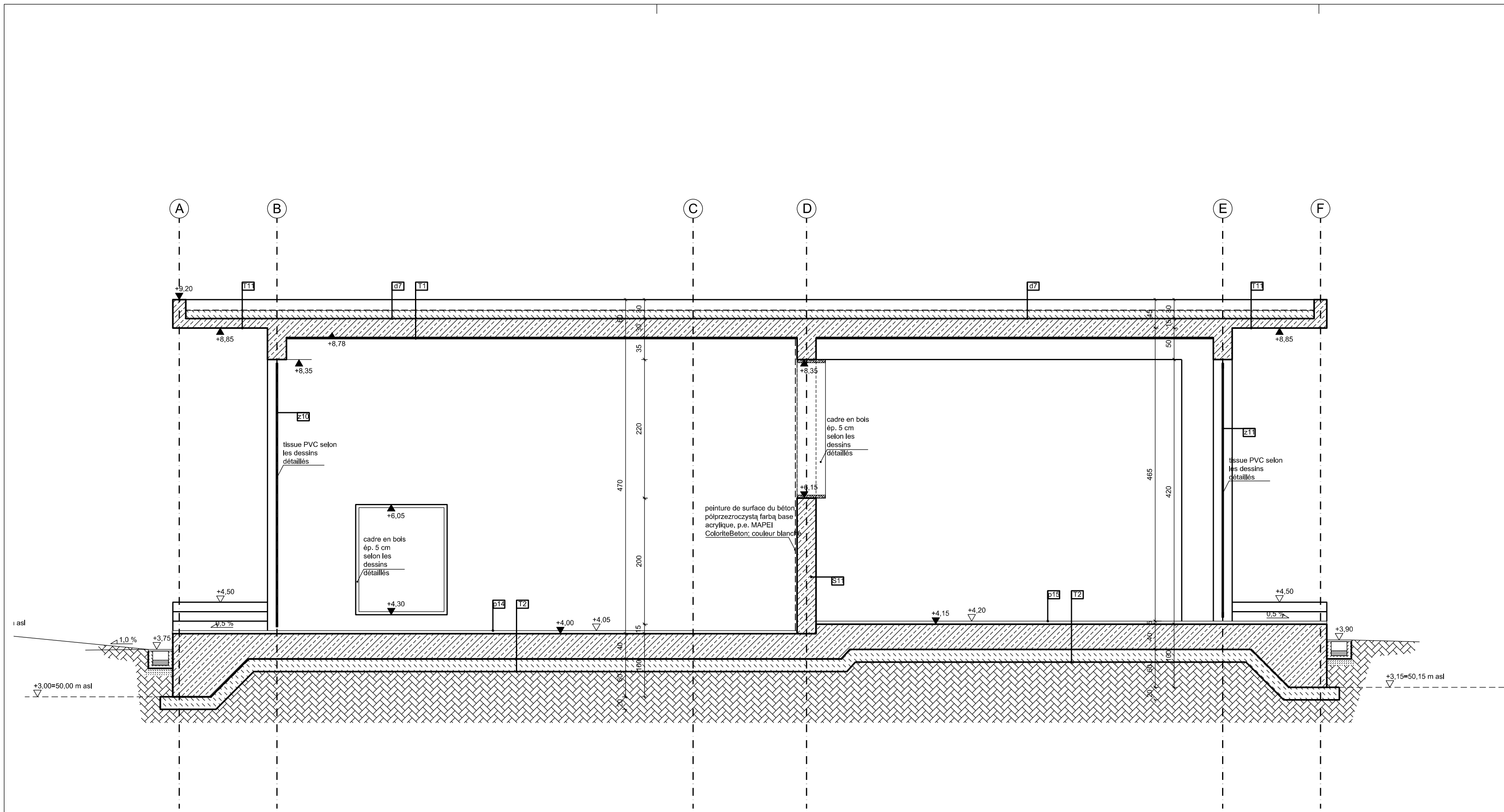
COUPE 19-20
