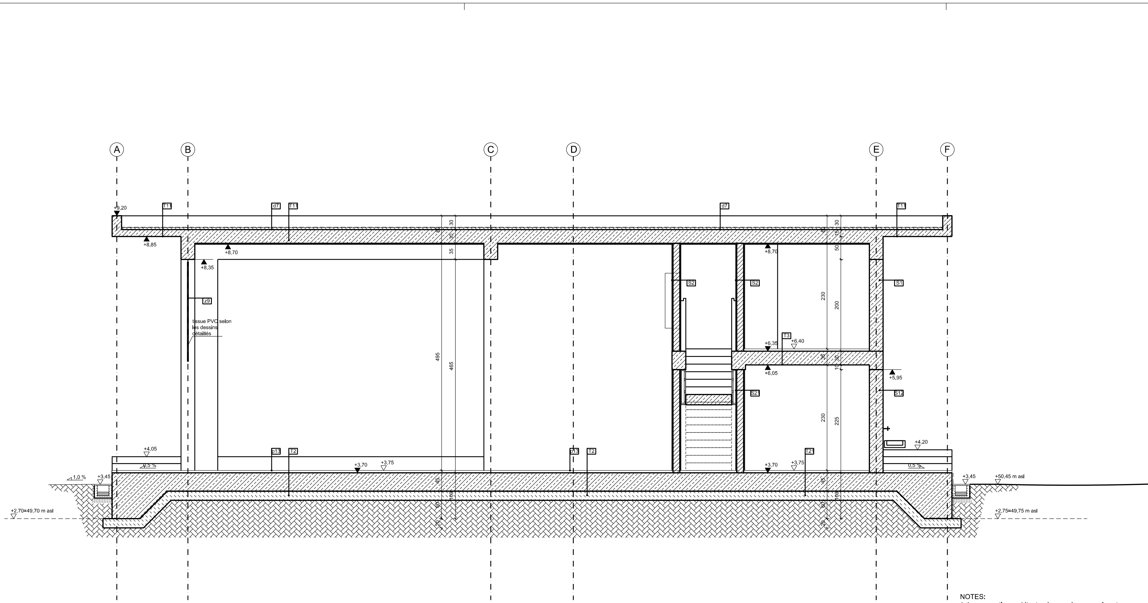
COUPE 17-18
