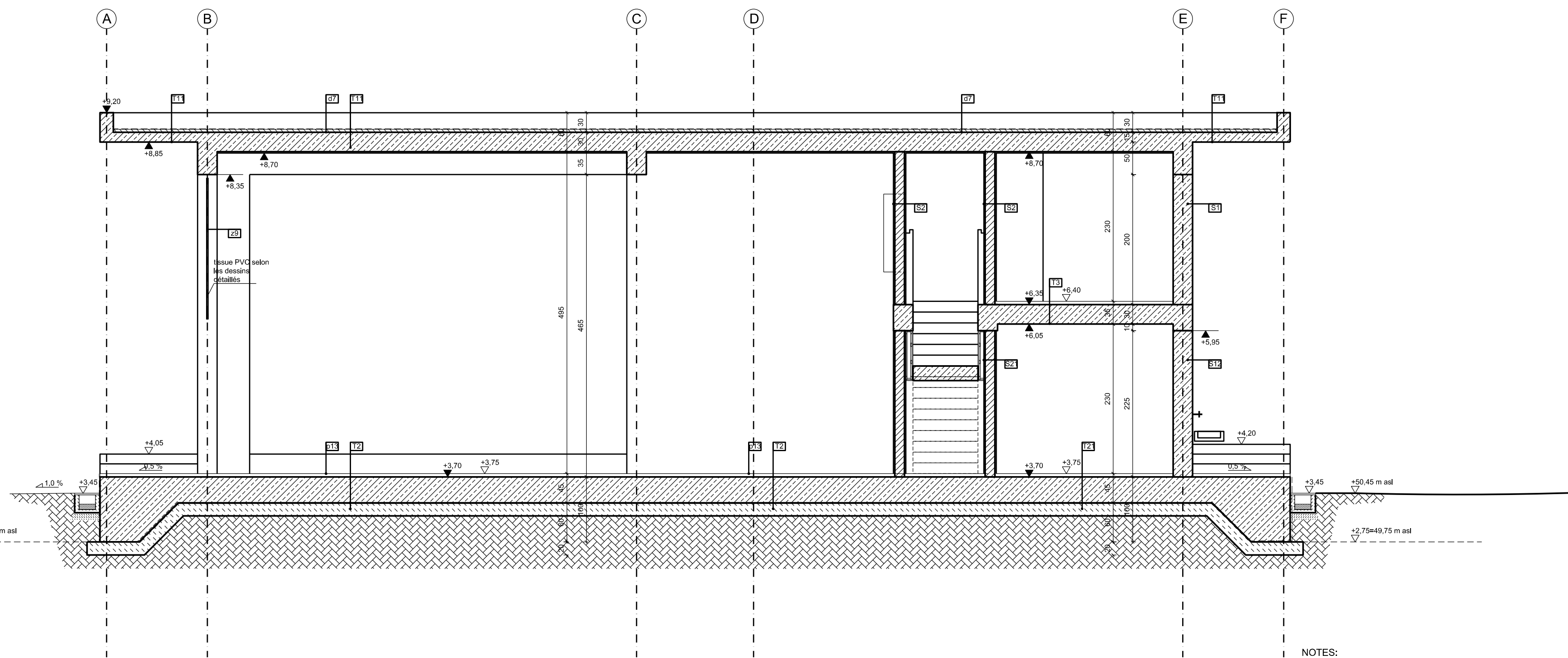
COUPE 17-18
