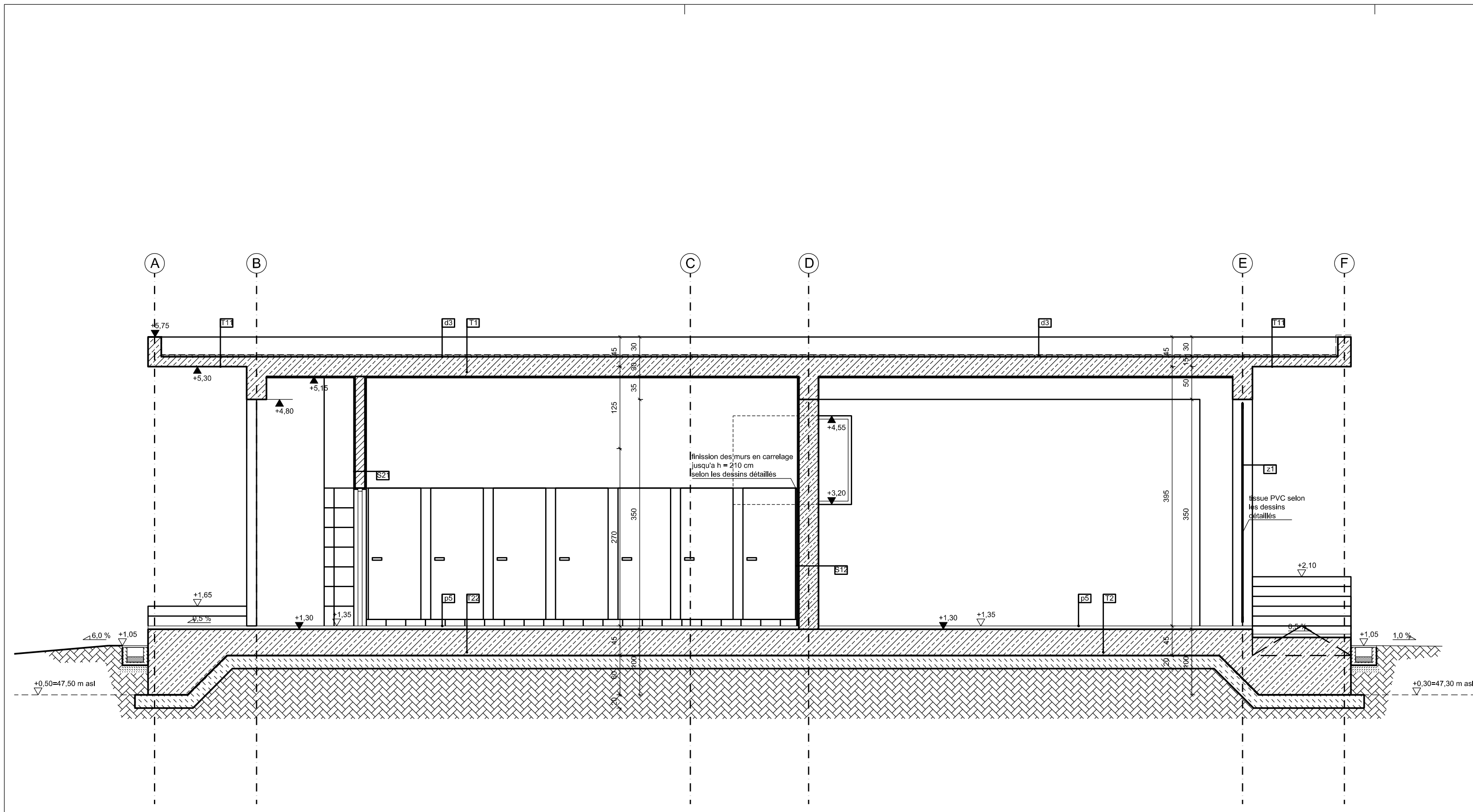
COUPE 7-8
