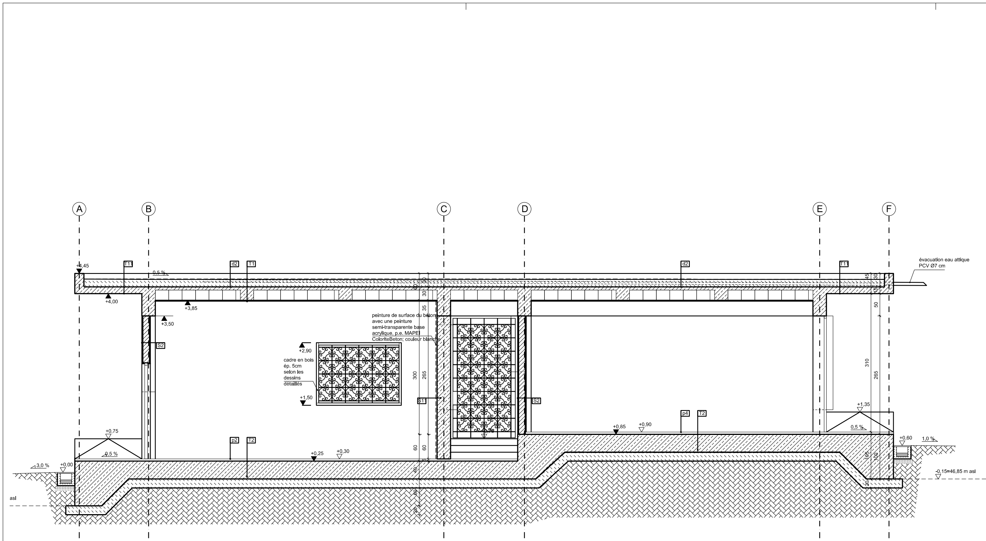
COUPE 3'-4
