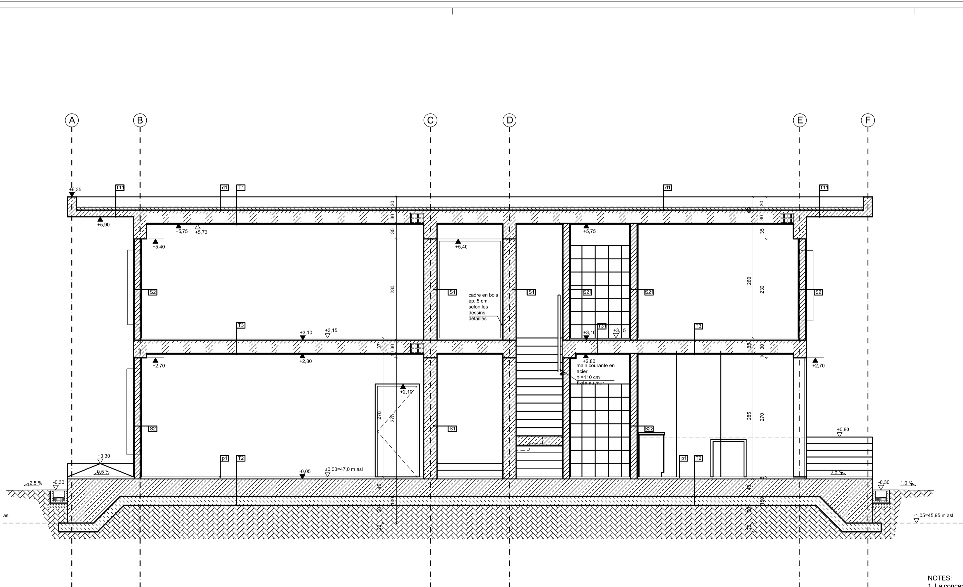
COUPE 1-2
